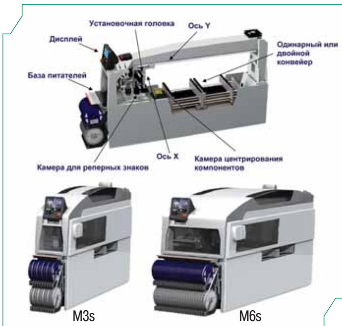
Рис.3 Установочные модули
