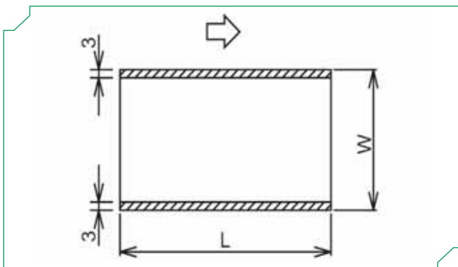
Рис.6 Необходимые свободные поля для фиксации платы на конвейере
